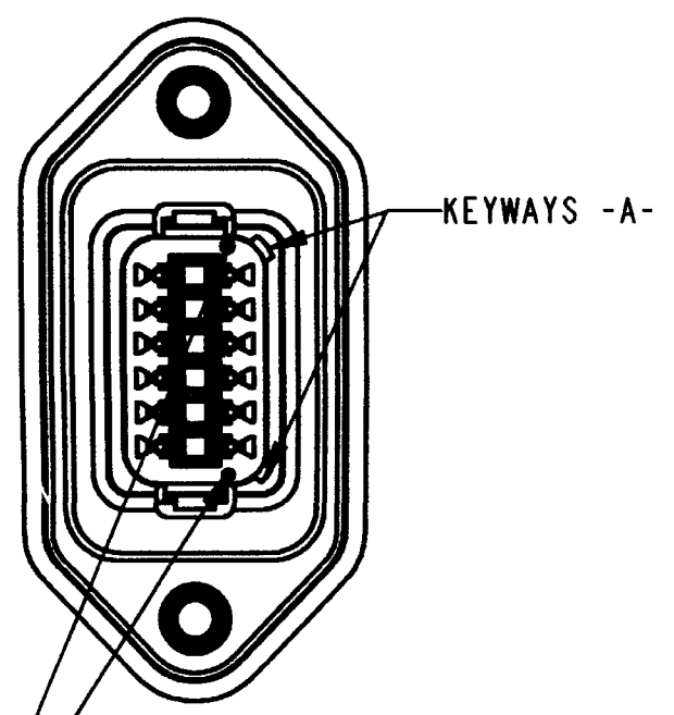
DT04-12PA-LE01 KEY ARR. -A- COLOR : GRAY
